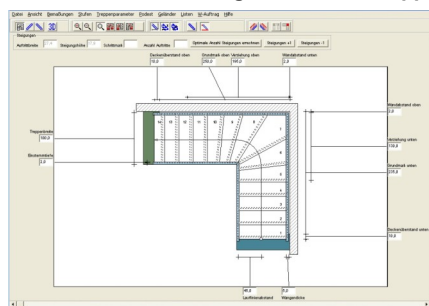
Draufsicht einer viertelgewendelten Treppe
