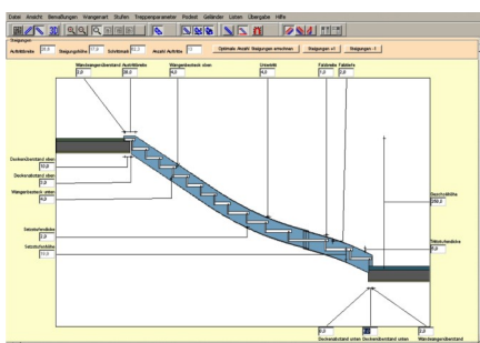
Wangenansicht einer viertelgewendelten Treppe
